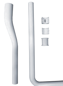
Tubo descarga ajustável Tubo de descarga ajustable Tadjustable flush pipe Tuyau de décharge coudé ajustable
