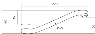
Bica inferior cromada Caño bajo cromo Low spout chromed Bec inférieure chrome
