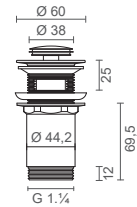
Tampão pequeno - aço inox · Tapa pequeña - acero inoxidable Small plug - stainless steel · Bouchon petit - acier inoxydable
